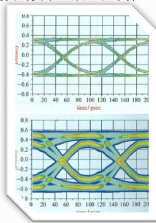
圖(三)訊號眼圖波形
