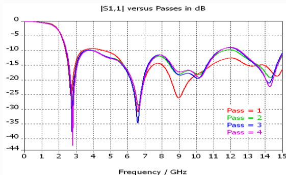
圖(五)為 ADS S_Paramter Simulation Result
