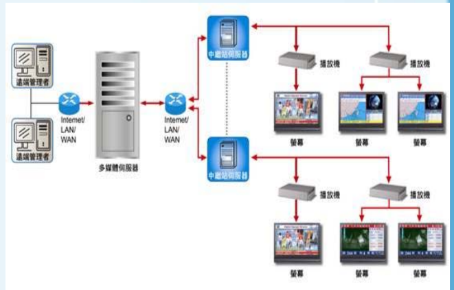
(圖二)多媒體系統網路架構圖
